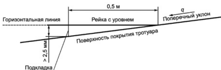
Рисунок 3 - Пример проверки поперечного уклона
